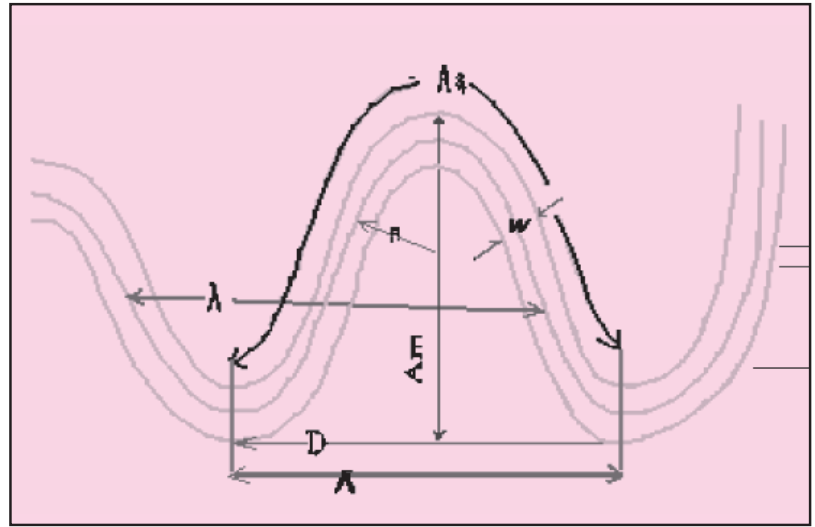
شکل ۲- متغیرهای مورفیک یک مئاندر
