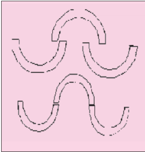
شکل ۱- مئاندرها به منزله نیمدایره‌های متوالی
