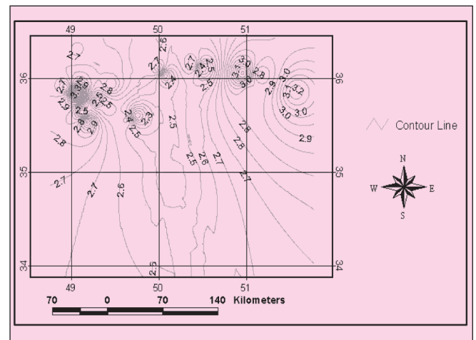
شکل ۴- نقشه ترسالی‌های شدید در طول دوره آماری مورد مقیاس زمانی ۶ ماهه
