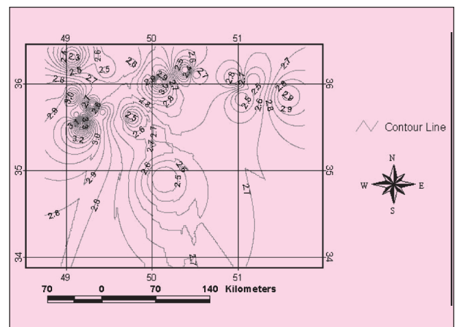
شکل ۶- نقشه ترسالی‌های شدید در طول دوره آماری مورد مطالعه در مقیاس زمانی ۱۲ ماهه
