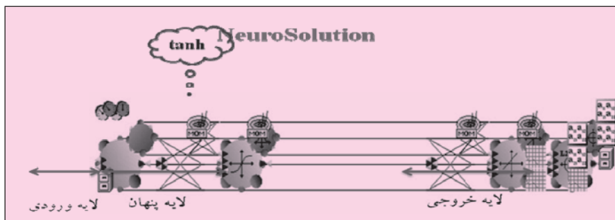
شکل ۲- مدل شبکه عصبی برای تعیین تابع تخمین کربن آلی خاک در نرم افزار NeuroSolution
