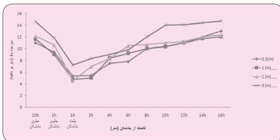
شکل شماره ۳- نمودار تغییرات طولی و ارتفاعی سرعت باد در اطراف بادشکن گزشاهی
