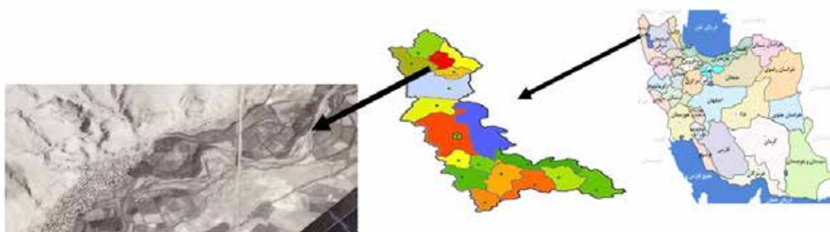
شکل ۱- نقشه موقعیت استان آذربایجانغربی در کشور و تصویر ماهواره ای محدوده مطالعاتی
