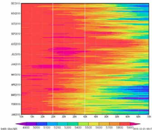
شکل ۶- هوف مولر برای تراز ۵۰۰ هکتوپاسکال سال ۲۰۱۰
