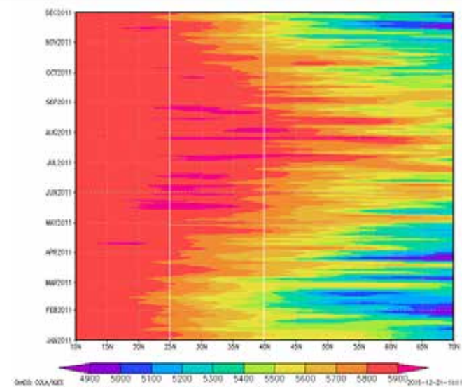
شکل ۵- هوف مولر برای تراز ۵۰۰ هکتوپاسکال سال ۲۰۱۱
