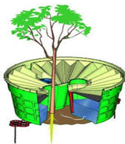
شکل ۱-۴۳- نمایی از واترباکس و نحوه عملکرد آن
